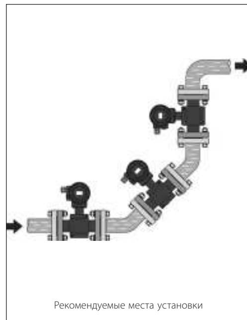
Установка в частично заполненных трубопроводах
